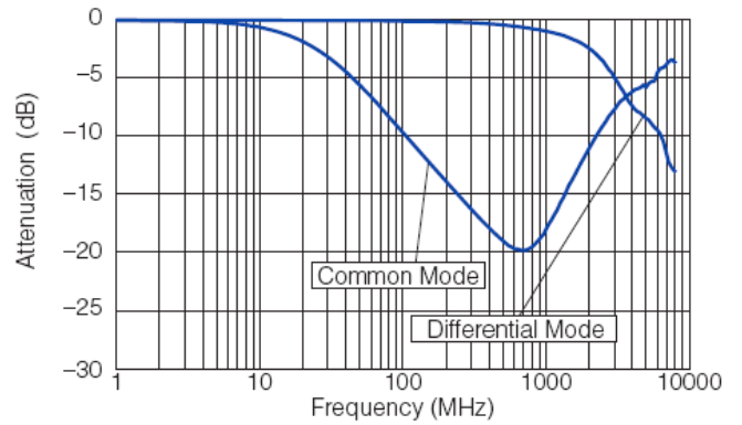
CMMC0806E121MST
