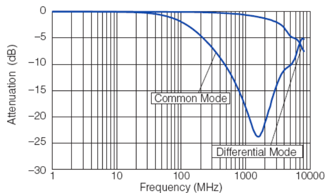
CMMC0806E350YST
