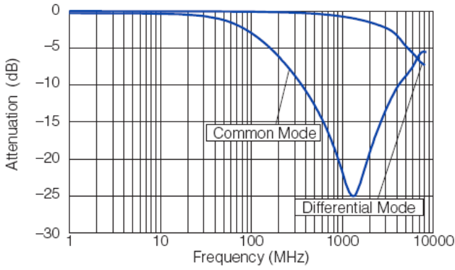
CMMC0806E450NST
