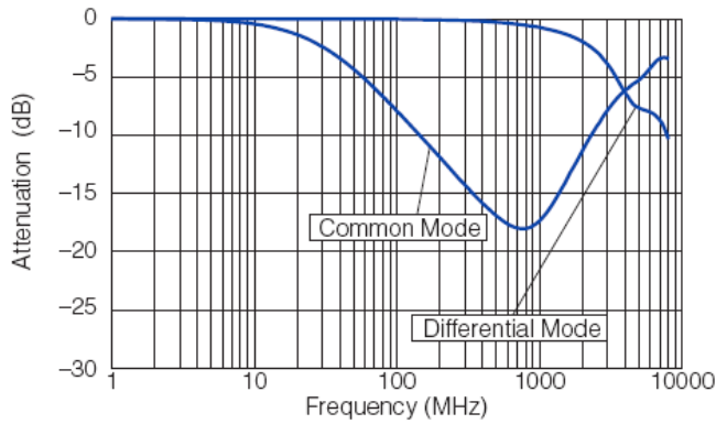
CMMC0806E900MST
