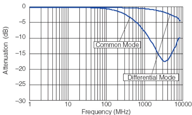
CMMC0806E120YST
