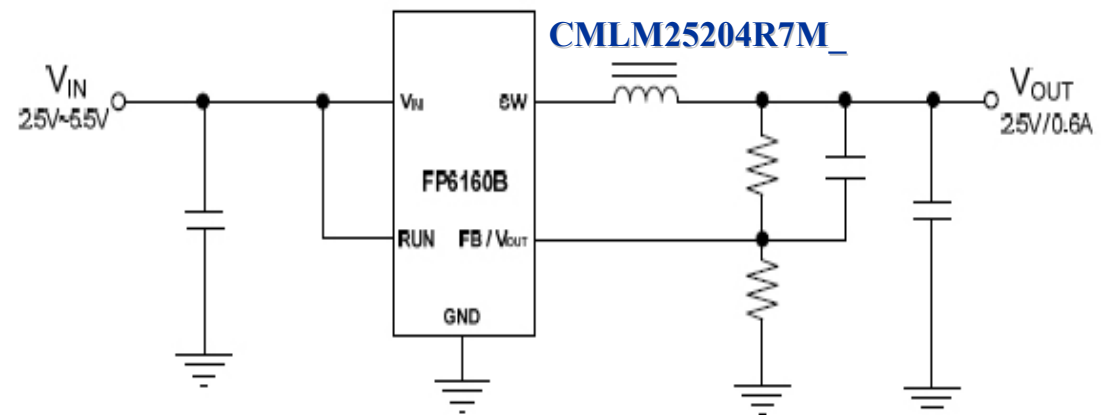
降压 (Buck)
